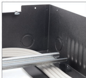
Szyny DIN na dystansie 27mm
