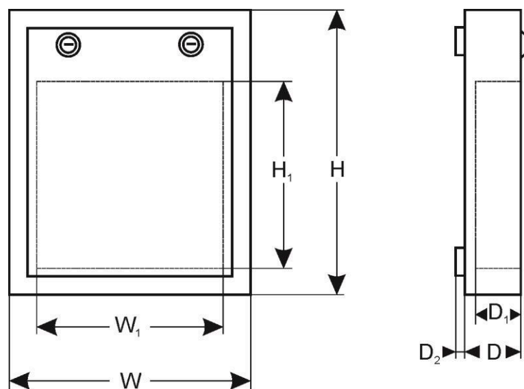
Obrázek 1. Rozměry.
