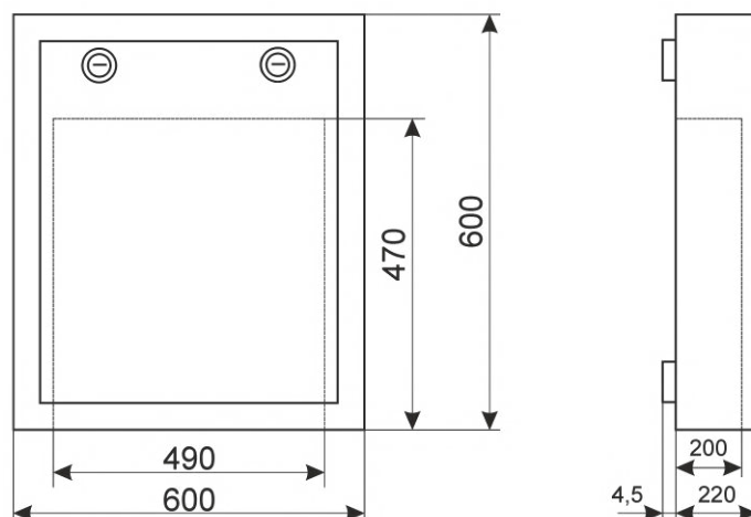
Rozměry.
