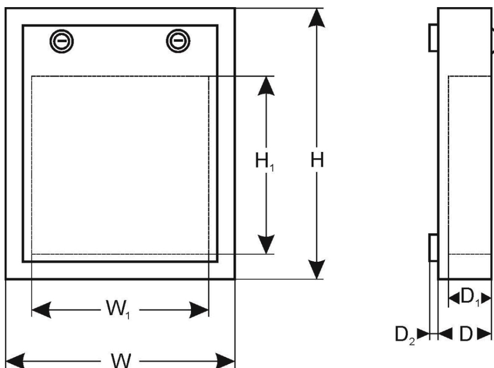
Rozměry.
