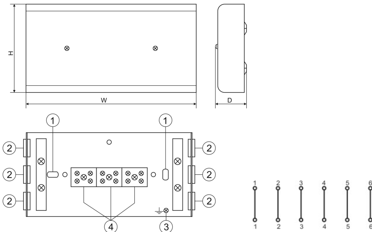
Obr. 1. Rozvodná skříň.
