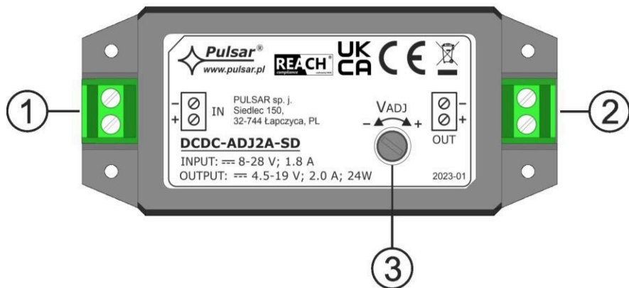
Obr. 2a. Pohled na modul měniče DCDC-ADJ2A-SD.
