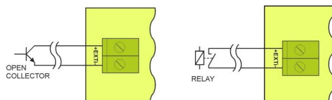
Obr. 6. Příklady zapojení.
