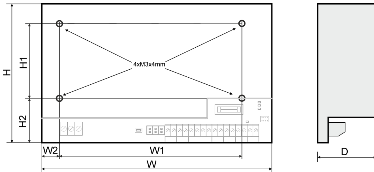
Obr. 3. Rozměry napájecí jednotky.
