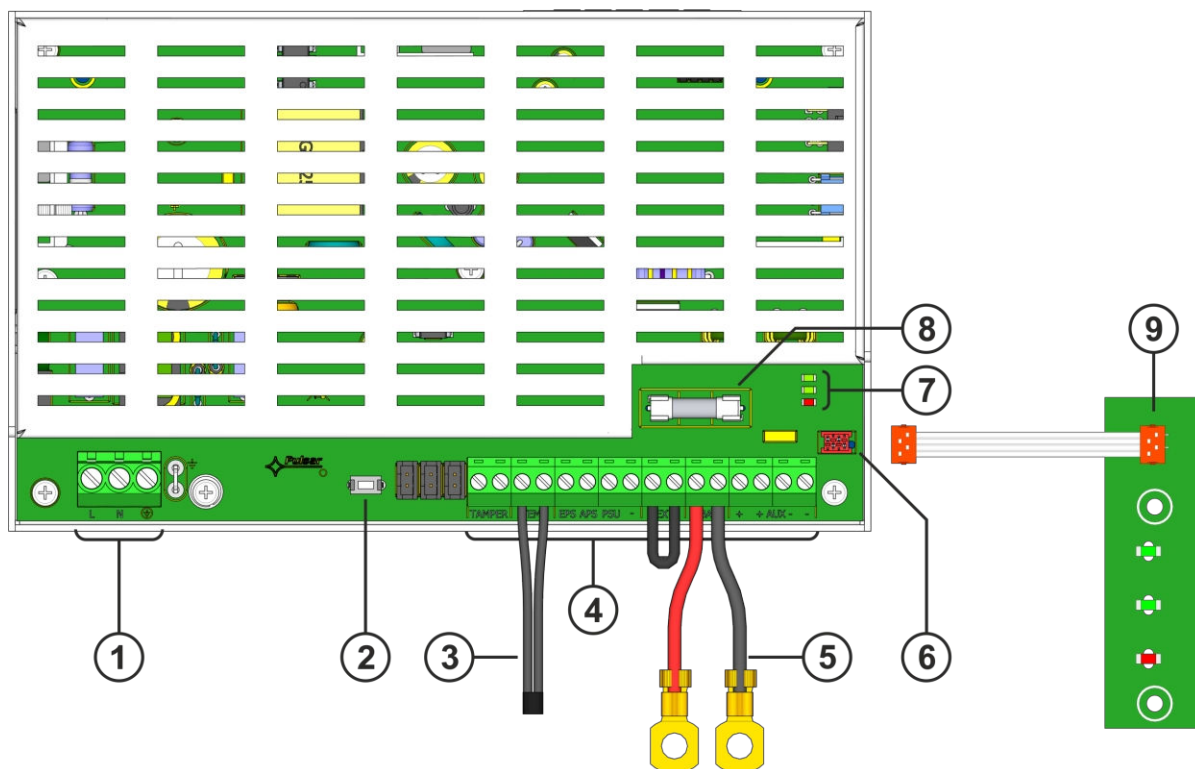
Obr. 2. Modul PSU.
