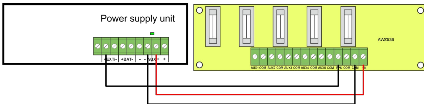
Obr. 7. Příklad zapojení s pojistkovým modulem AWZ536.
