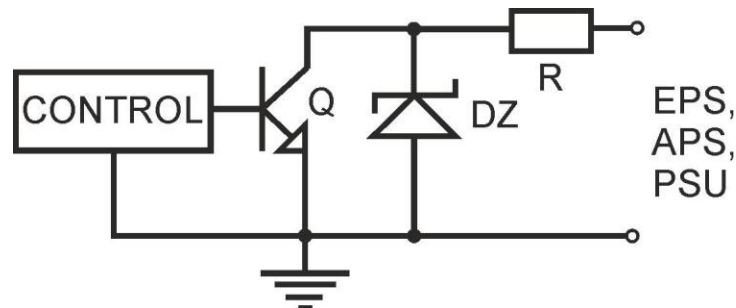
Obr. 4. Elektrické schéma technických výstupů.
