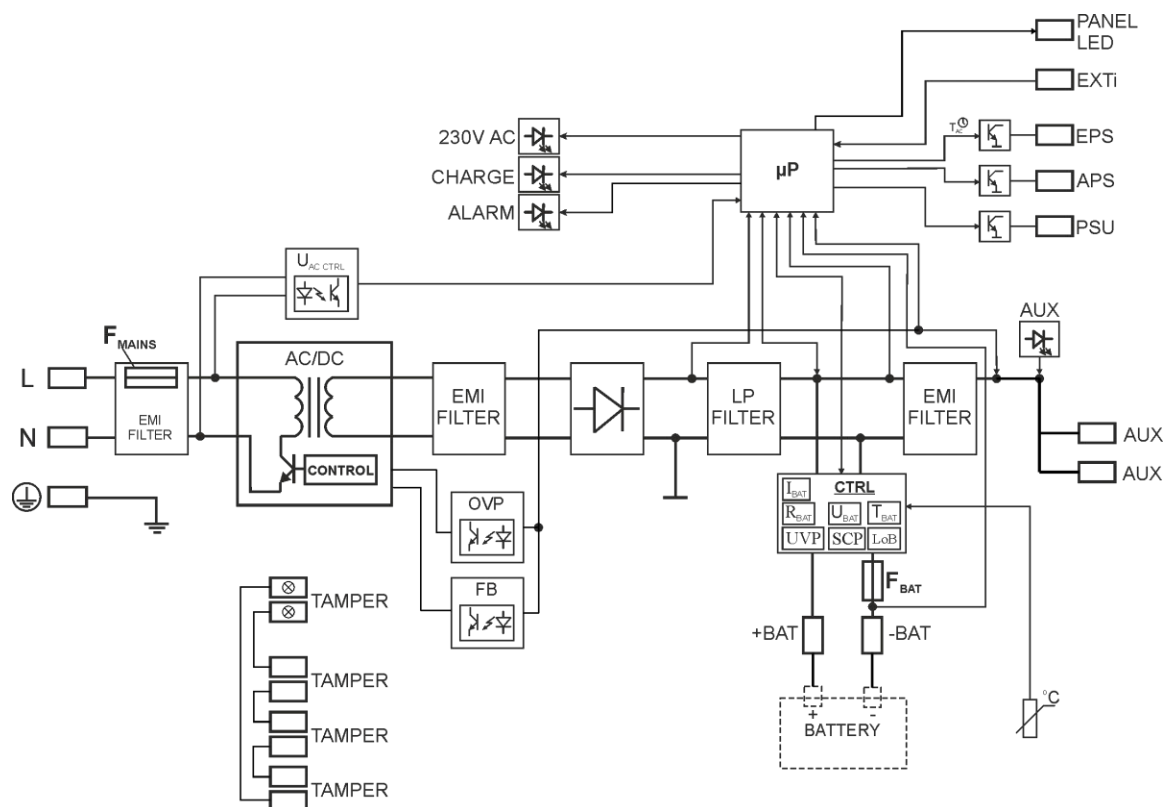
Obr. 1. Blokové schéma PSU.
