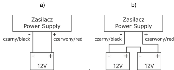
Obr. 4 Připojení baterií v závislosti na napěťové verzi zdroje:
