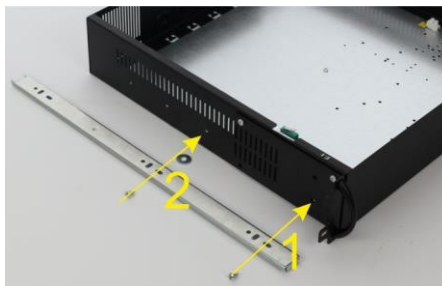
Befestigen Sie die Schieber mit zwei Schrauben am ARAD-Gehäuse (die Distanzscheibe unter der zweiten Schraube nicht vergessen)
