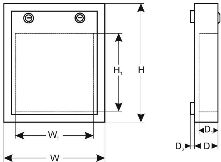
Abbildung 1. Abmessungen.
