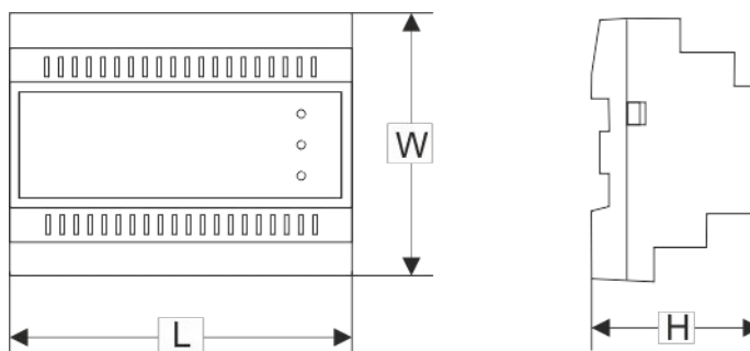
Abb. 2b. Ansicht des Stromversorgungsmoduls (Modelle 12V3A, 12V5A, 24V2A, 24V3A)
