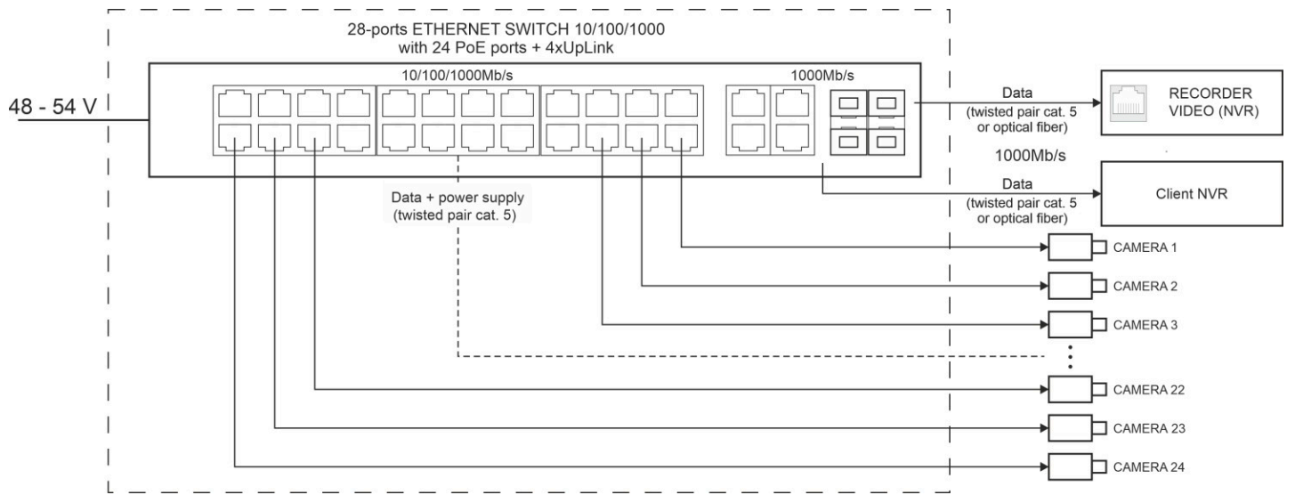
Abb. 1. Blockdiagramm.
