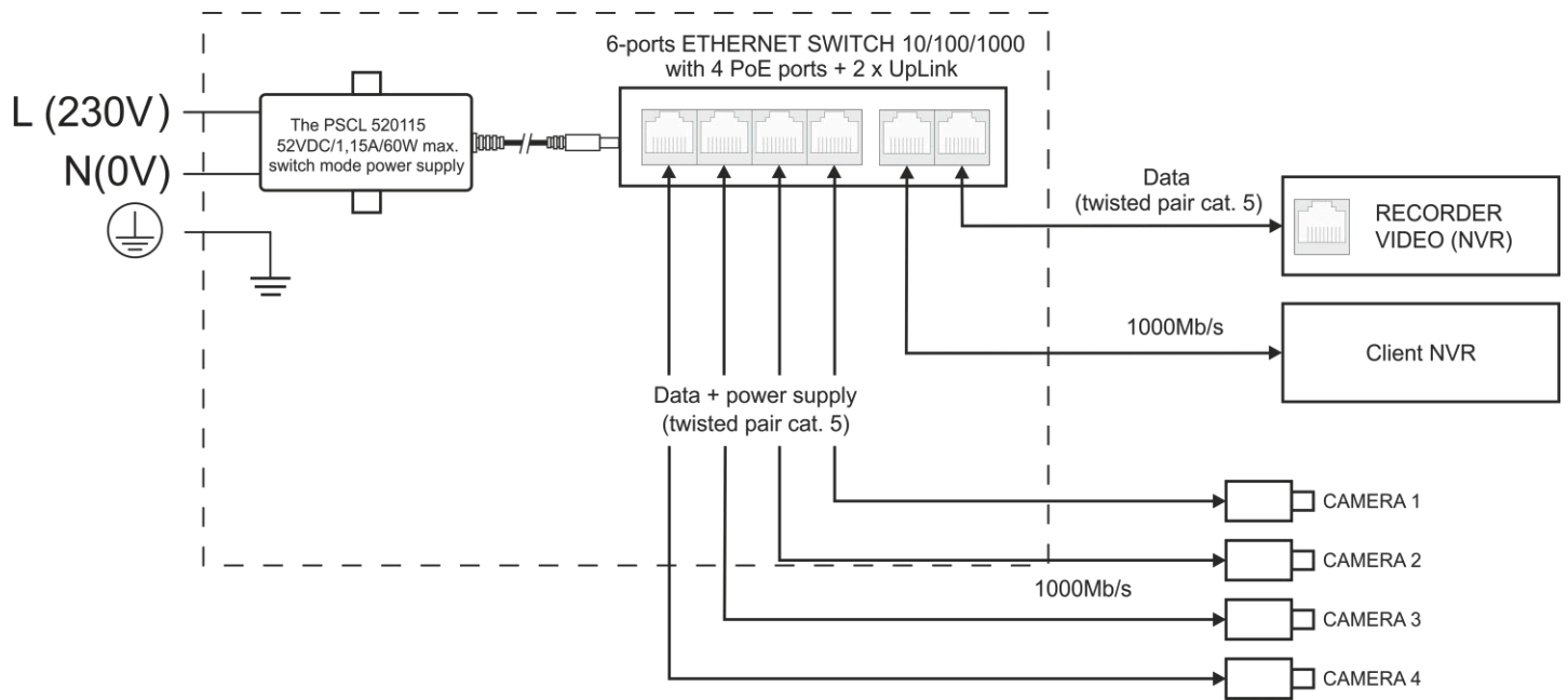
Abb. 1. Blockdiagramm.
