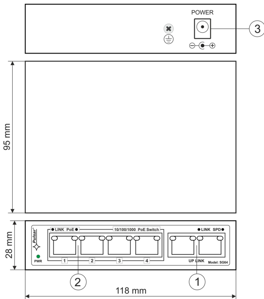
Abb. 3. Ansicht des Schalters a.
