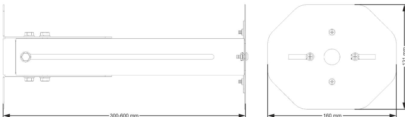
Fig. 1. Dimensions
