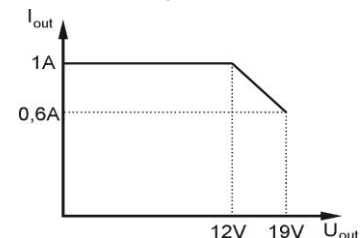
Fig.3. Corriente máxima de salida dependiendo del voltaje de salida.
