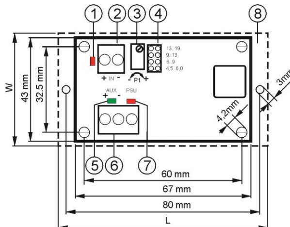
Fig.2. Vista del módulo del convertidor.
