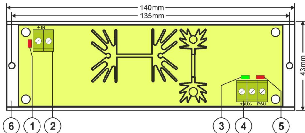
Fig.2. Vista del módulo del convertidor.
