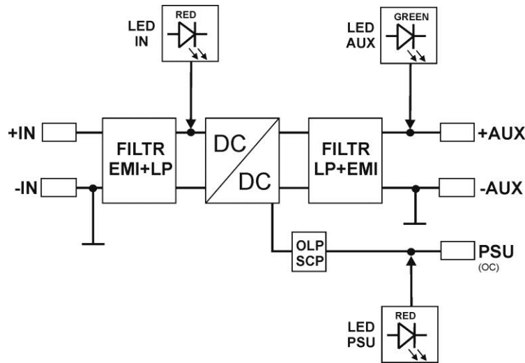
Fig.1. Esquema de bloques del módulo del convertidor.
