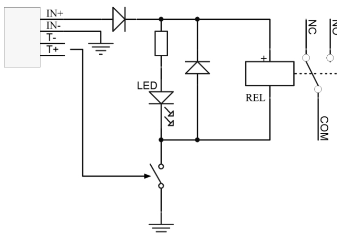
Fig. 2. Schéma électrique.
