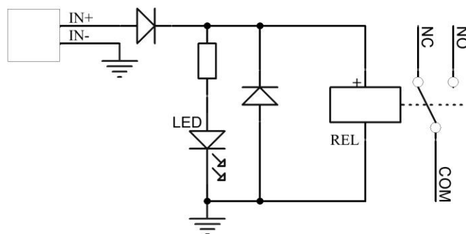
Fig. 2. Schéma électrique.
