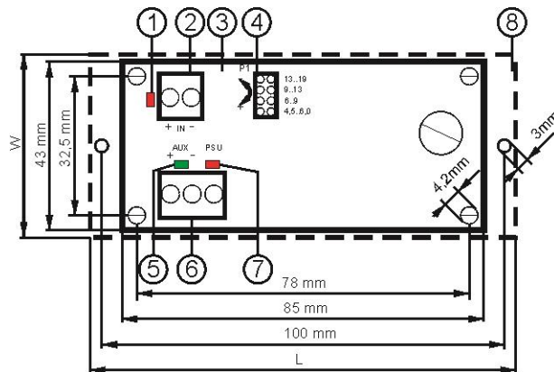
Σχ.2. Κάτοψη μονάδας μετατροπείας.
