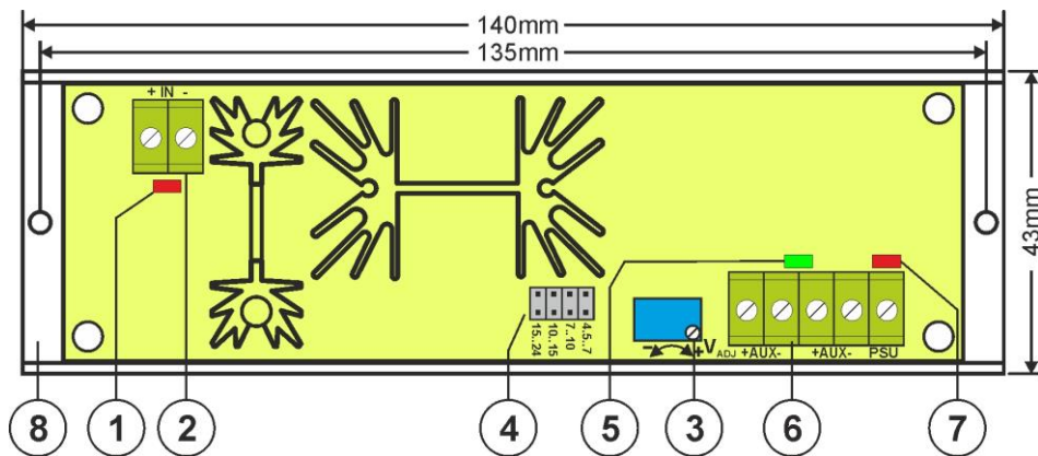
Σχ.2. Κάτοψη μονάδας μετατροπέα.
