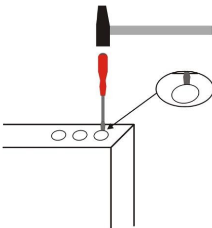
Εικ. 4. Η μέθοδος διαμόρφωσης ενός ανοίγματος για στυπιοθλίπτη καλωδίου.
