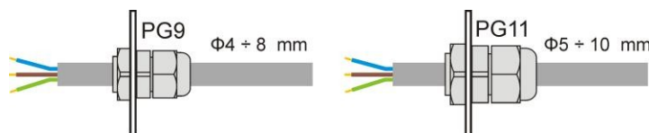
Εικ. 5. Συνιστώμενοι τύποι και διατομές καλωδίων εγκατάστασης PG9 και PG11 για καλωδιακούς σφιγκτήρες.
