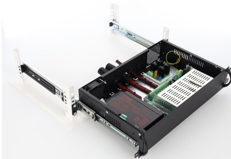
Csúsztassa a burkolatot a csúszkákkal együtt a 19 hüvelykes RACK szekrénybe szerelt sínekbe
