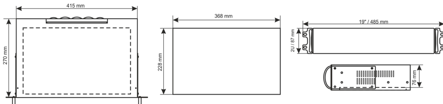
2. ábra: Méretek.
