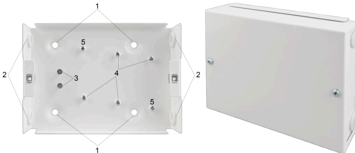
1. ábra: A hangszóróvonal-felügyeleti rendszer burkolatának nézete.
