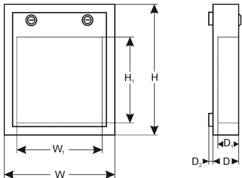
1. ábra. Méretek.
