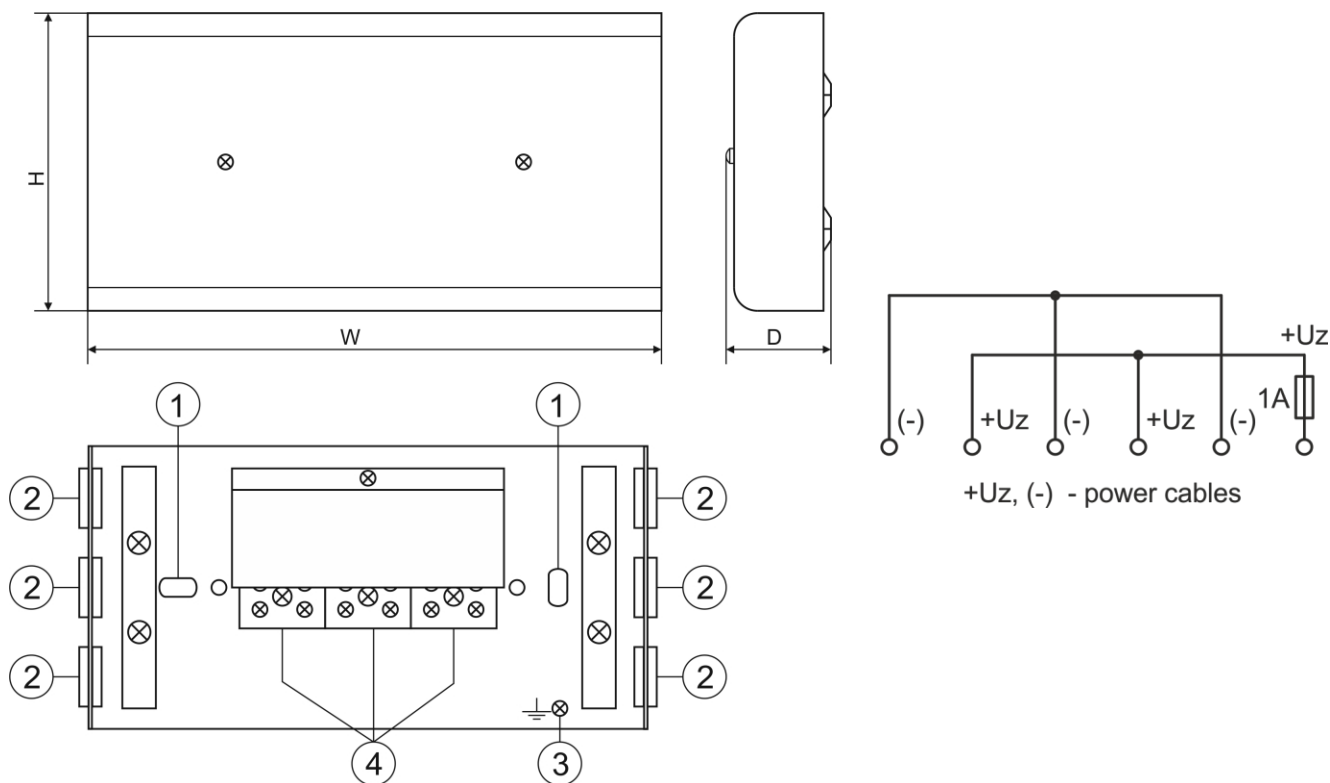
1. ábra. A csatlakozódoboz és a kapcsolási rajz.
