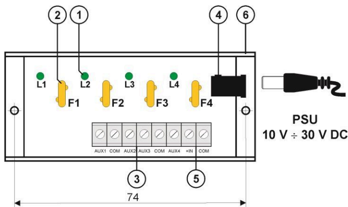
1. ábra: A modul rajza.
