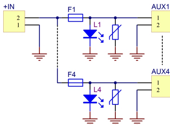
2. ábra: Elektromos kapcsolási rajz
