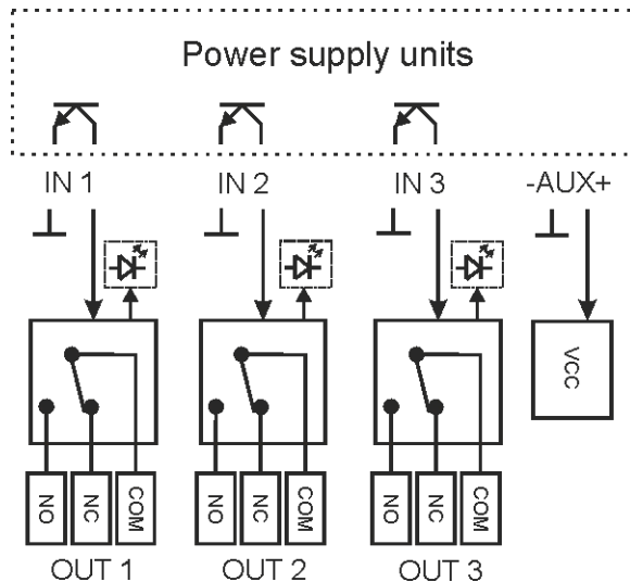
2. ábra. Blokkvázlat.
