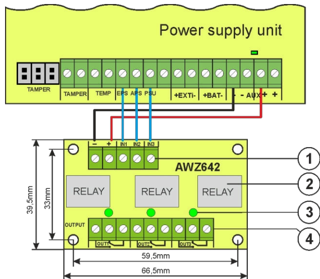
1. ábra. A modul sémája.
