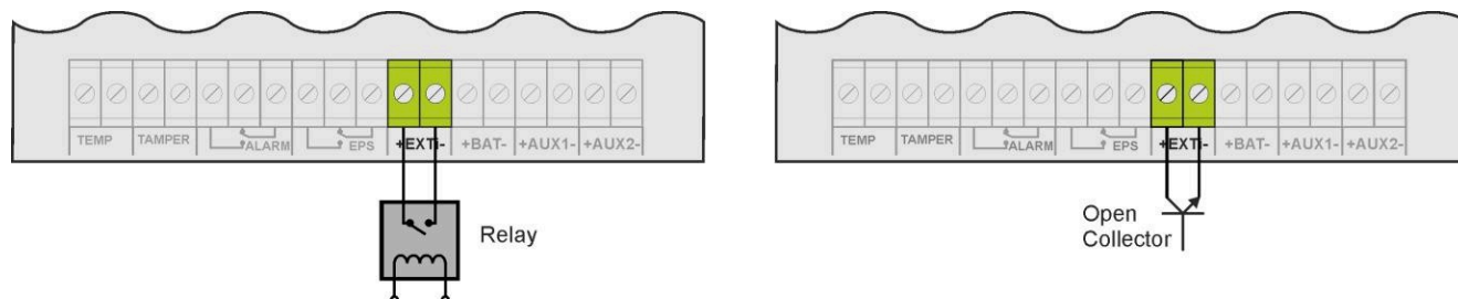
10. ábra. Csatlakozások az EXTi bemenethez.
