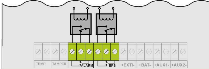
7. ábra. A relé kimenetek elektromos kapcsolási rajzai.
