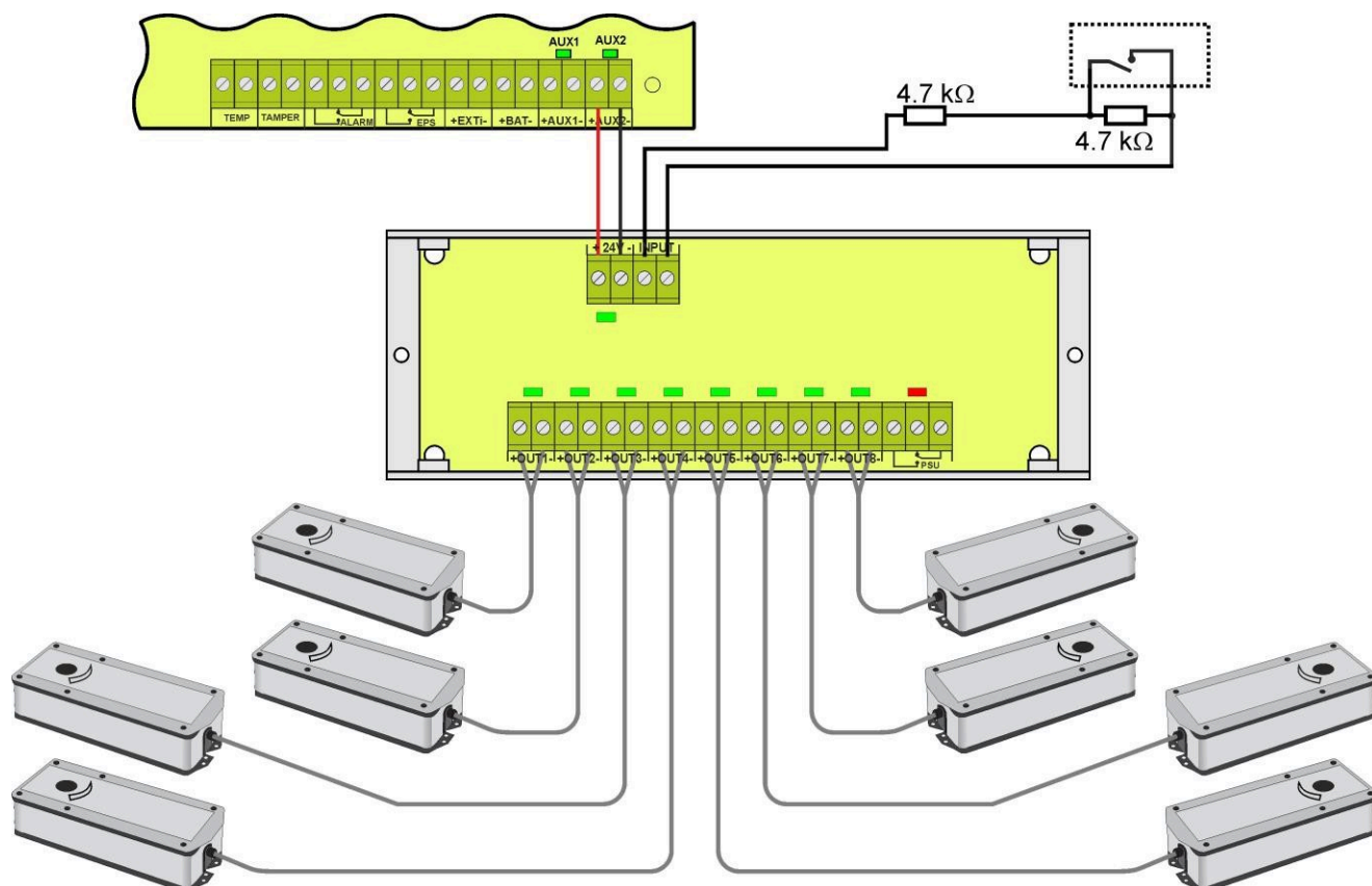
13. ábra. Példa az EN54C-LS8 szekvenciális modul csatlakoztatására a visszatérő rugóval ellátott működtetőikkel.
