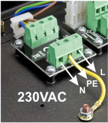
Scheda di alimentazione PCB in un alloggiamento
