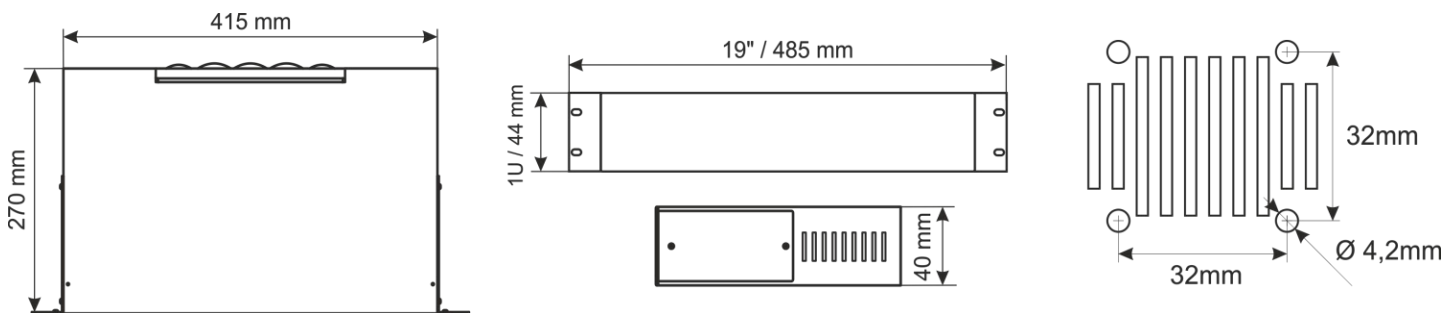
Figura 2. Dimensioni.
