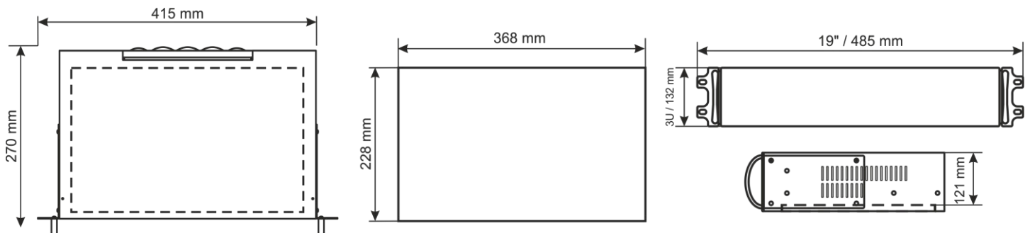
Figura 2. Dimensioni.
