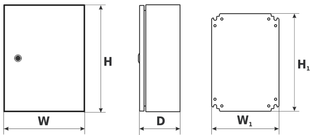
Fig. 2. Dimensioni.
