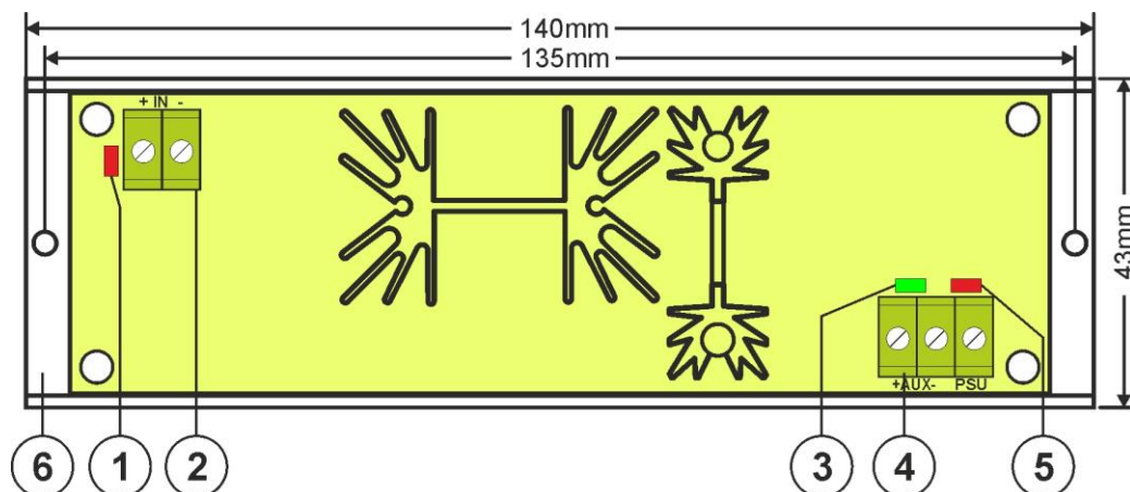
Fig.2. Vista del modulo del trasformatore.
