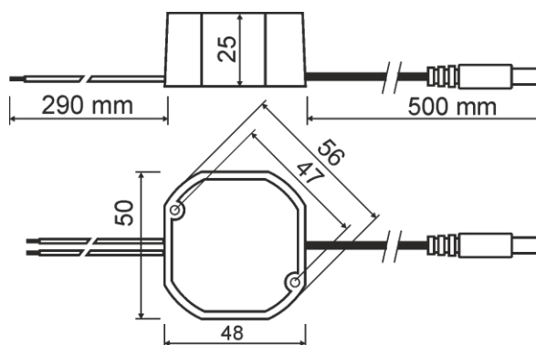
Fig. 1. Vista meccanica e dimensioni del convertitore.
