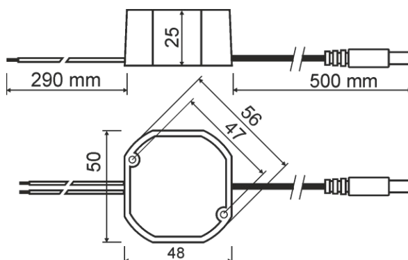
Fig. 1. Vista meccanica del convertitore.
