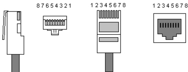
Fig. 3. Vista di un connettore RJ-45.
