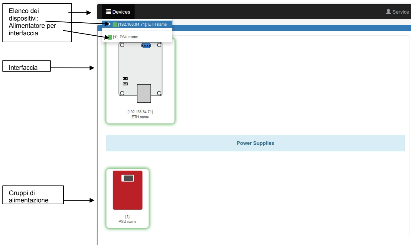
Fig. 21. Vista della scheda "Dispositivi".
