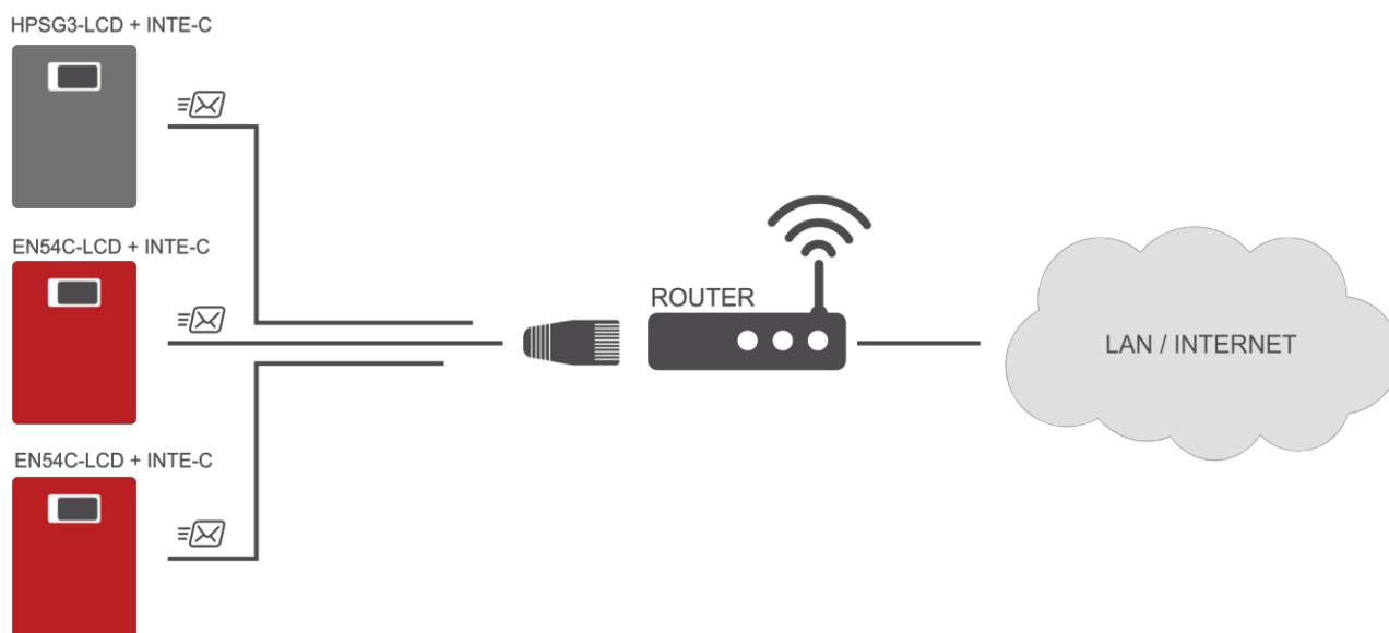
Fig. 1. Schema di principio della comunicazione in rete Ethernet.
