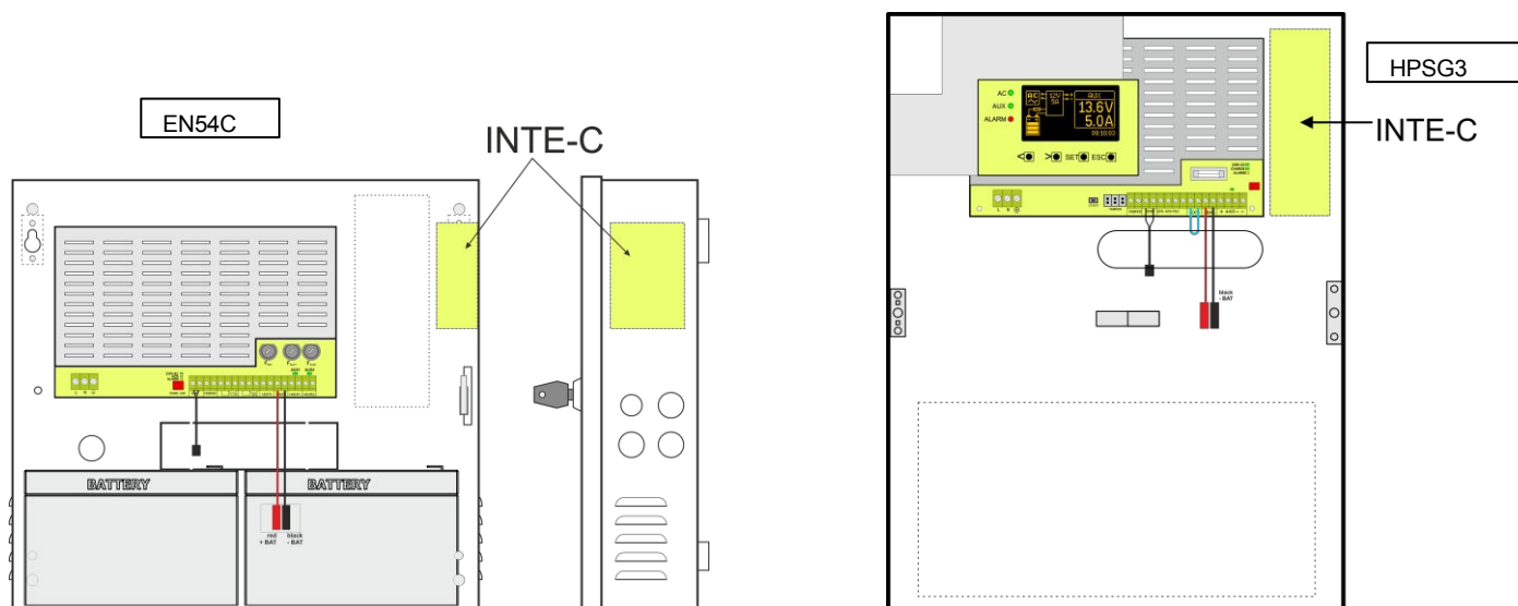
Fig. 4. Posto di installazione indicato dell'interfaccia INTE-C.
