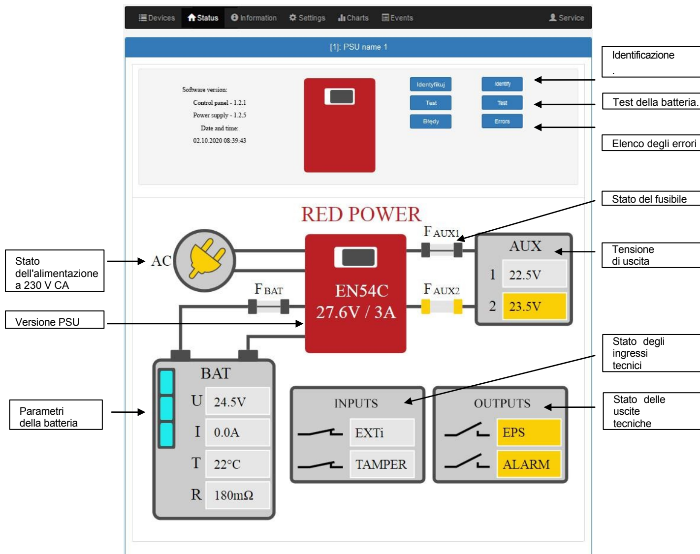
Fig. 10. Vista della scheda "Stato" della serie di alimentatori EN54C-LCD.
