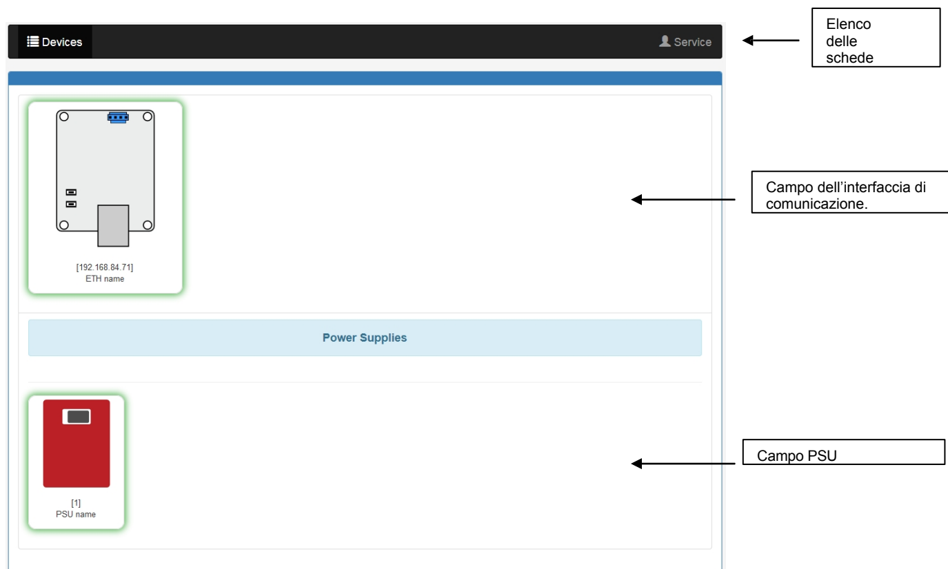
Fig. 8. Vista della scheda «Dispositivi» – connessione con alimentatore serie EN54C.
