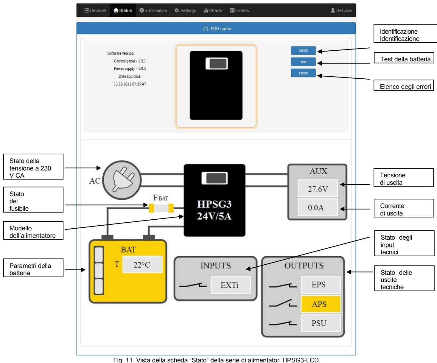
Fig. 11. Vista della scheda "Stato" della serie di alimentatori HPSG3-LCD.
