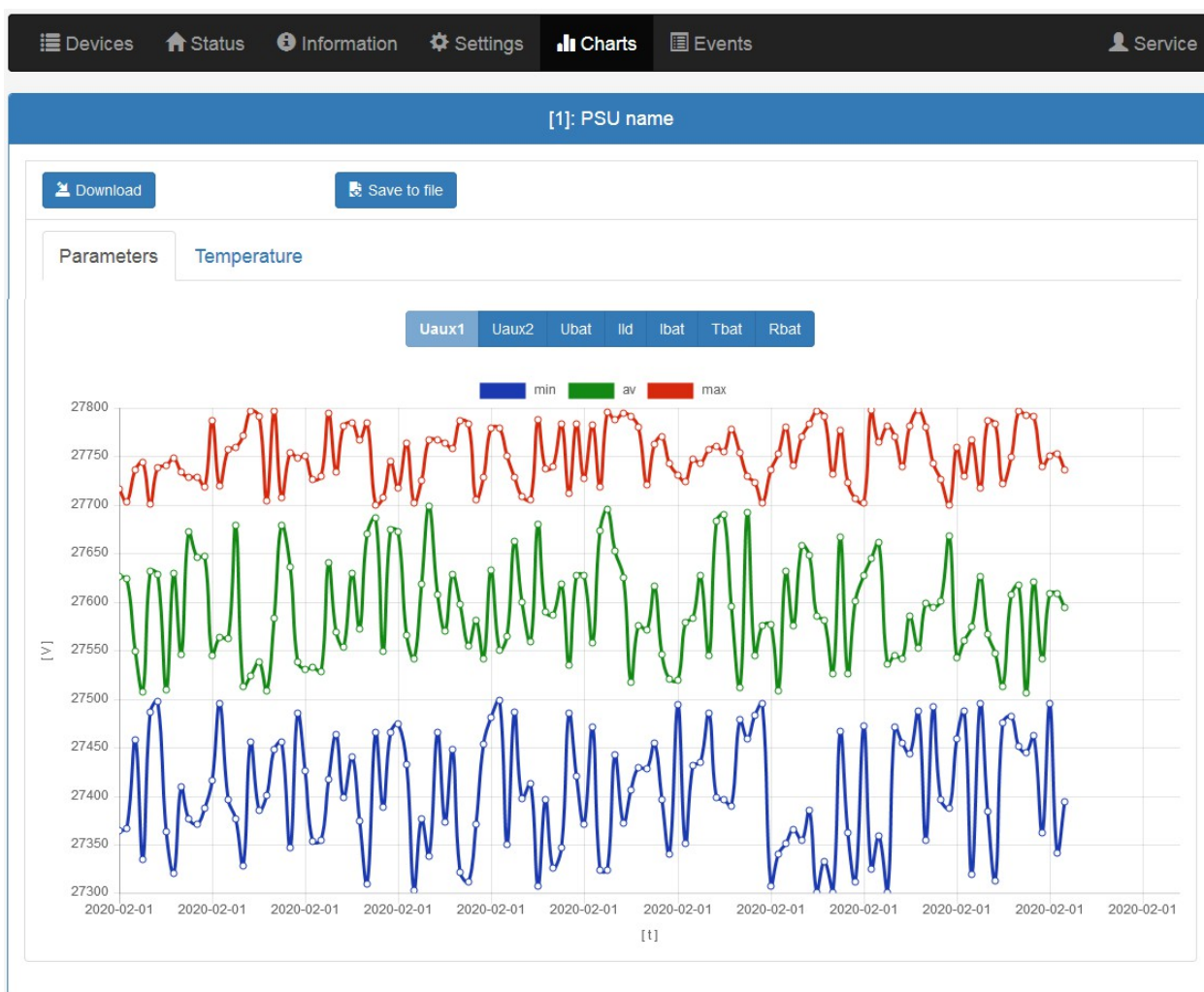
Fig. 19. Grafico di esempio dei parametri, rilevati dall'alimentatore EN54C-LCD.
