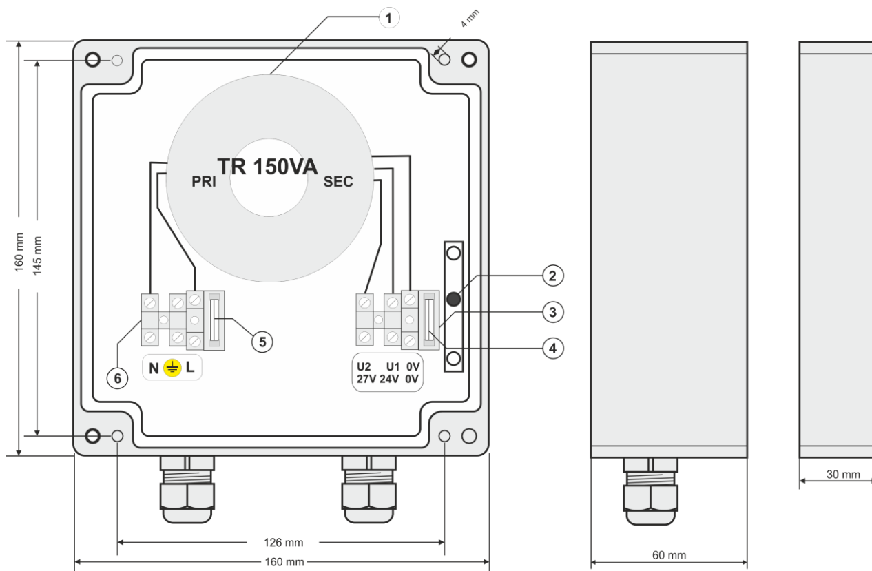
Fig.2. Vista dell'alimentatore.
