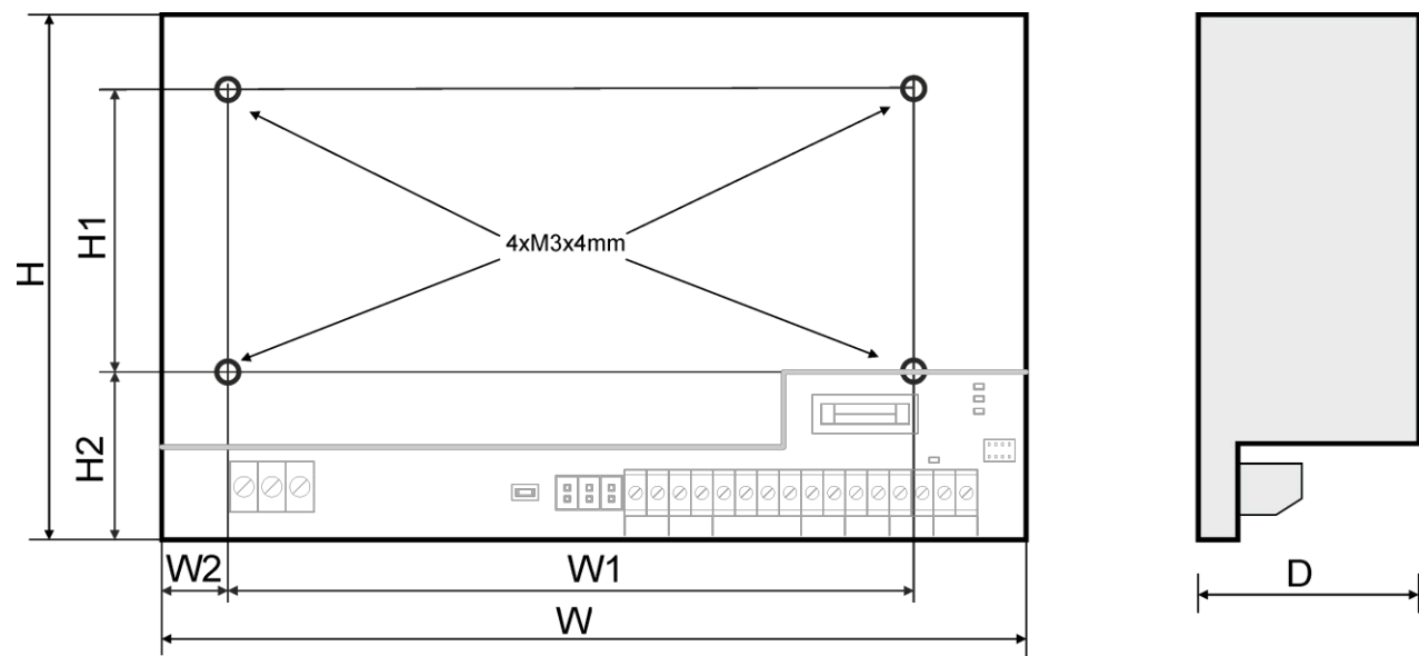
Fig. 3. Dimensioni dell'alimentatore.
