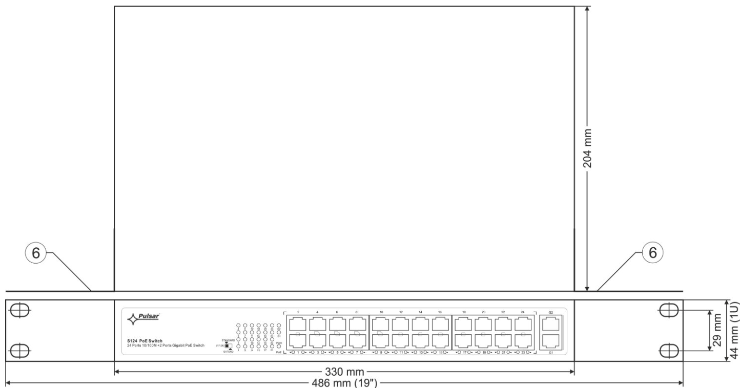
Fig. 4. Vista del commutatore.
