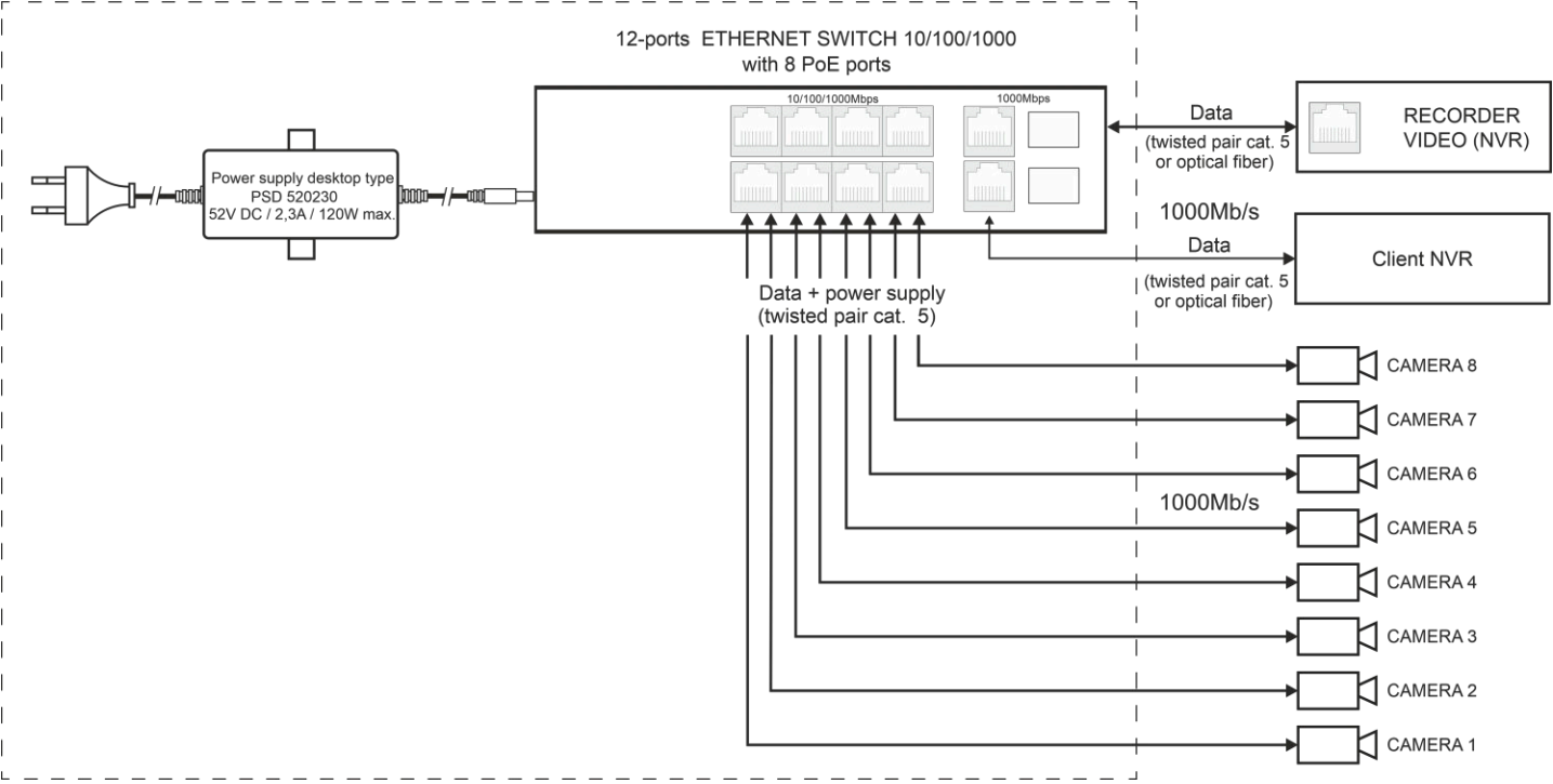
Fig. 1. Schema a blocchi.
