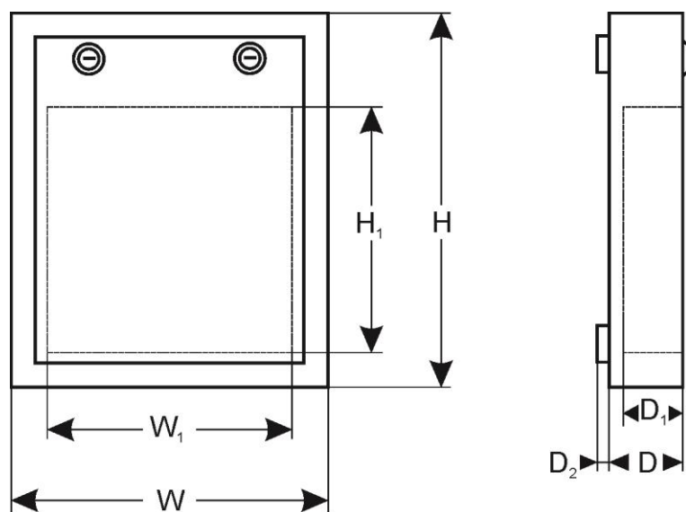
Rysunek 1. Wymiarowanie.
