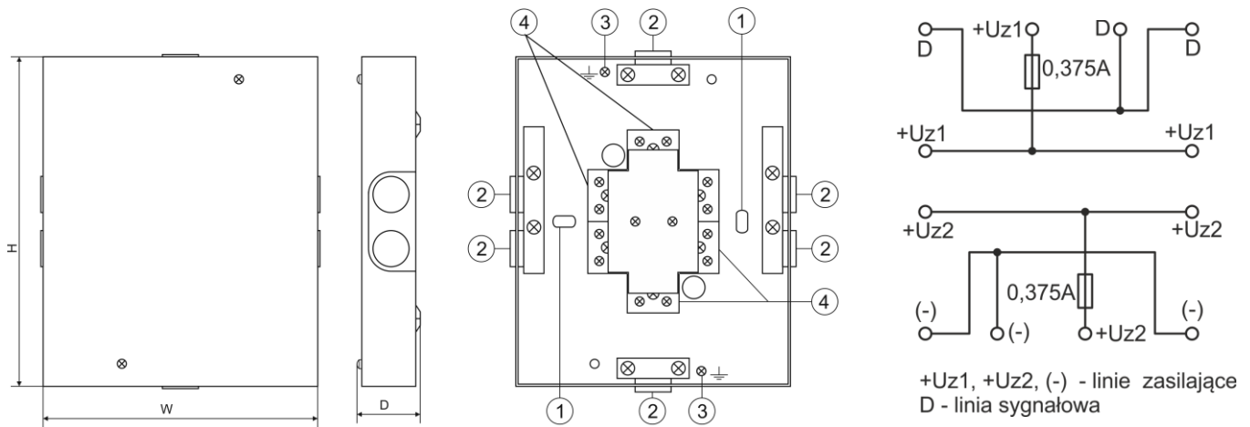
Rys.1. Widok puszk instalacyjnej i schemat połączeń.
