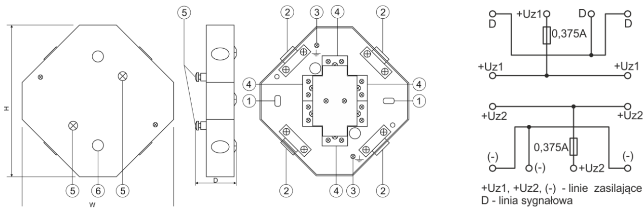
Rys.1. Widok puszek instalacyjnych i schemat połączeń.
