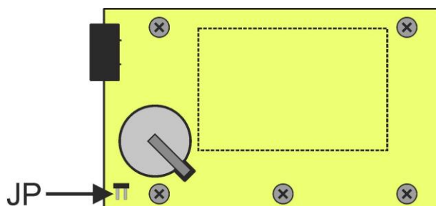
Rys. 29. Lokalizacja zworki JP na płycie PCB wyświetlacza.
