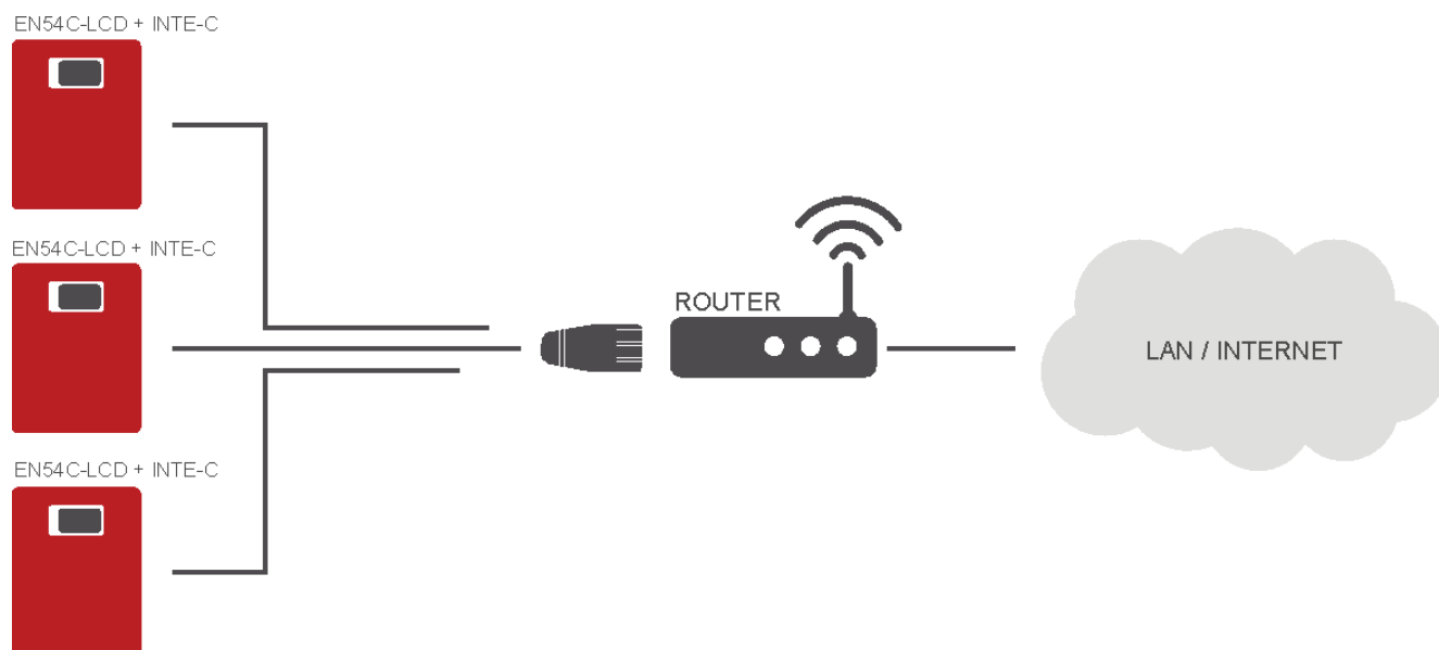
Rys. 32. Komunikacja Ethernet z wykorzystaniem interfejsu „INTE-C”.
