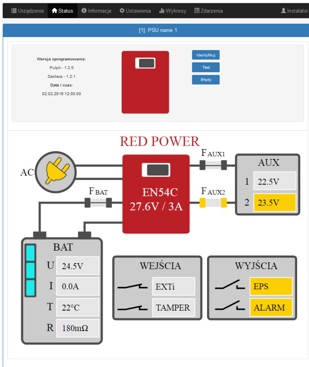
Rys. 34. Widok stanu zasilacza.
