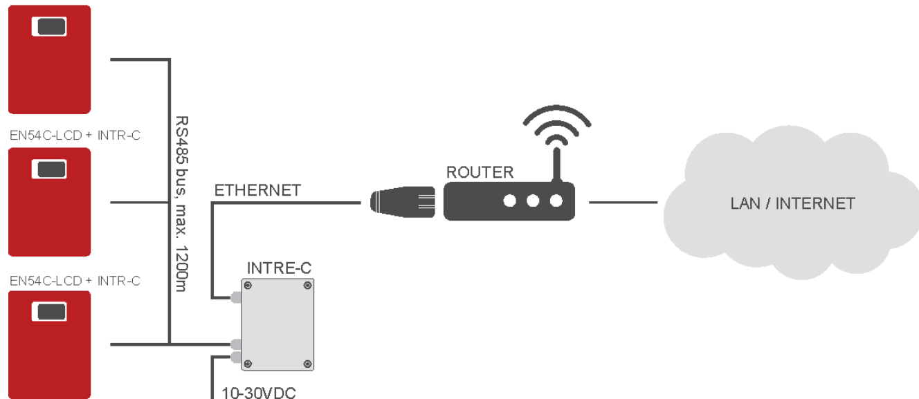
Rys. 33. Komunikacja Ethernet z wykorzystaniem interfejsów „INTR-C” oraz „INTRE-C”
