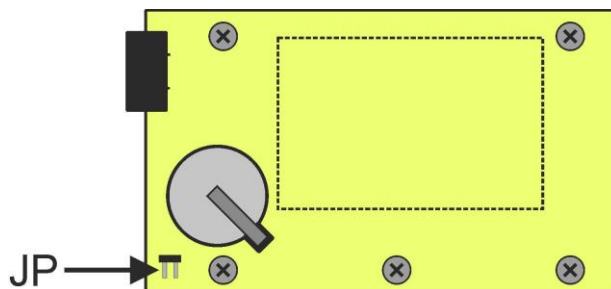
Rys. 25. Lokalizacja zworki JP wykorzystywanej w procedurze odblokowywania haseł.
