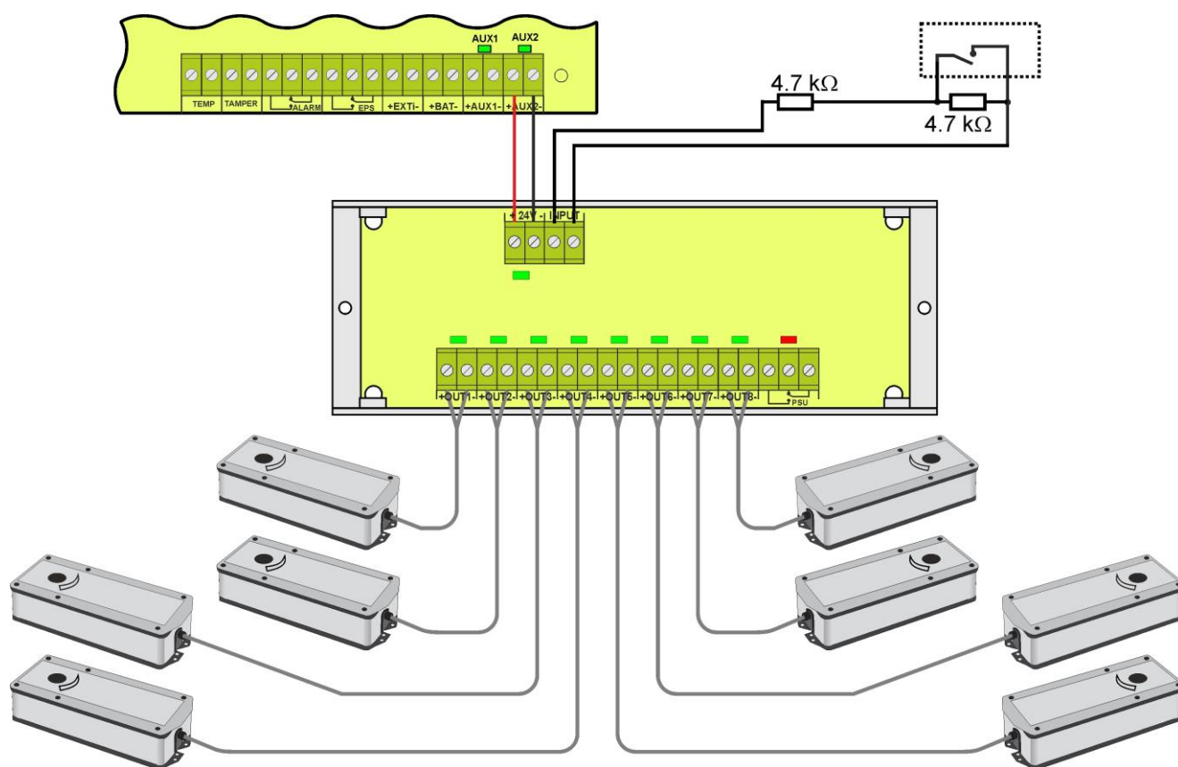
Rys. 12. Przykładowy sposób podłączenia z modulem sekwencyjnym EN54C-LS8 i siłownikami ze sprężyną powrotną.
