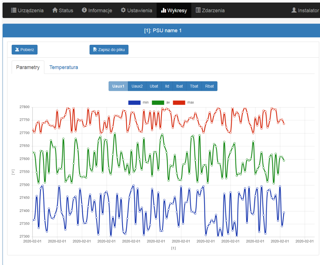
Rys. 35. Widok historii pracy zasilacza.
