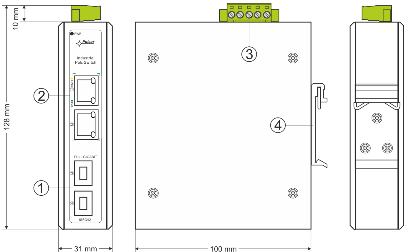
Rys. 2. Widok switch'a.
