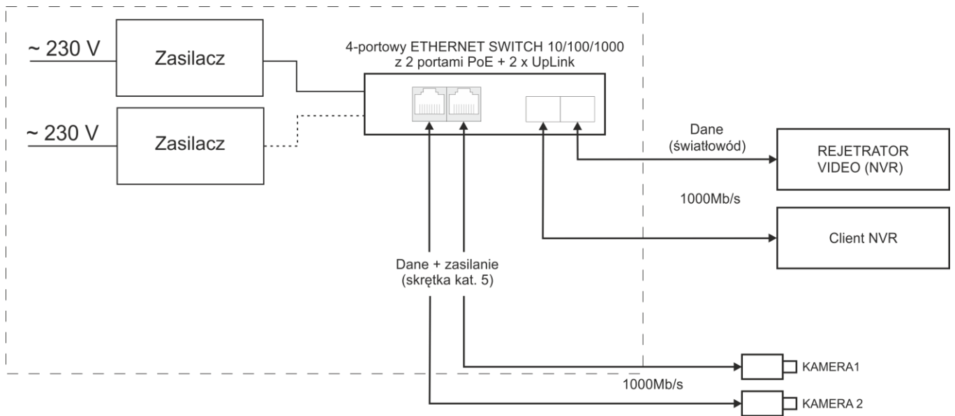
Rys. 1. Schemat blokowy.
