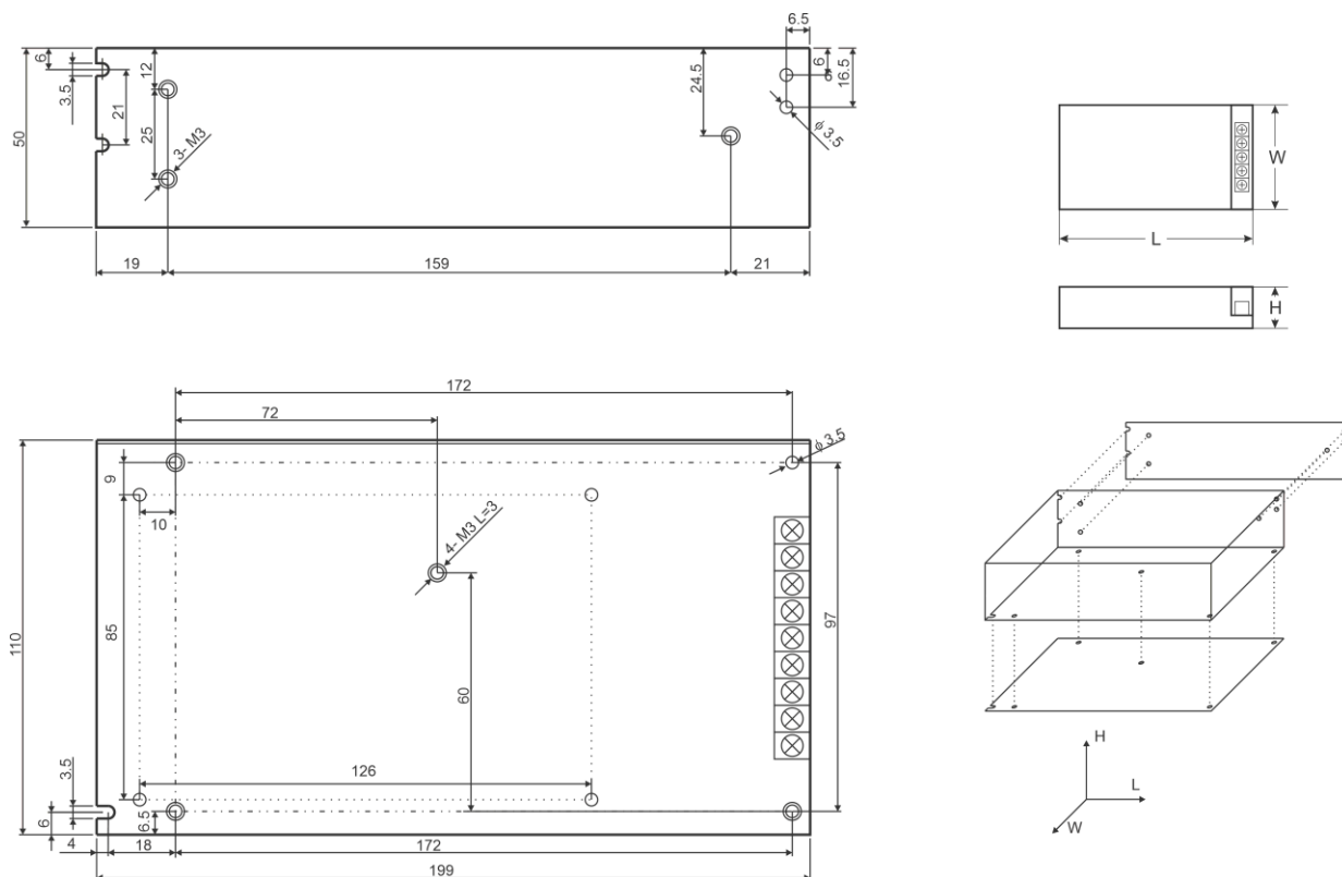
Rysunek 2. Widok mechaniczny zasilacz
