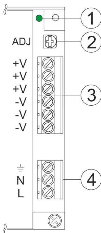
Rysunek 1. Opis złącz zasilacza.
