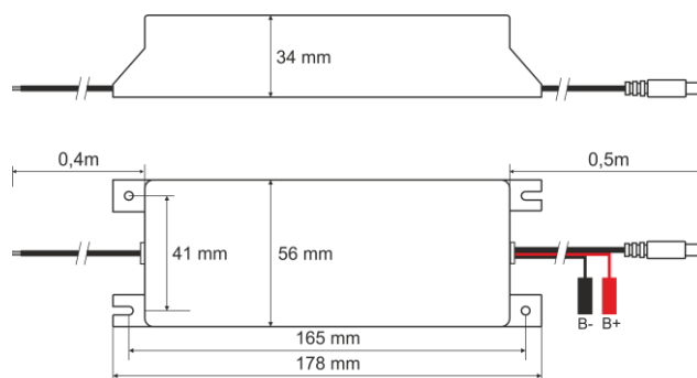
Rys.1. Widok mechaniczny zasilacza.
