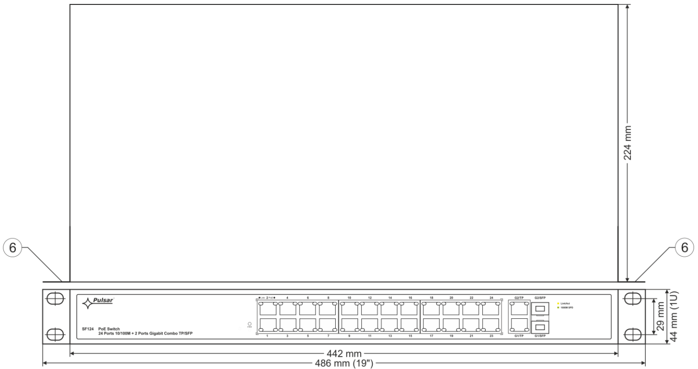
Rys. 4. Widok switch'a.
