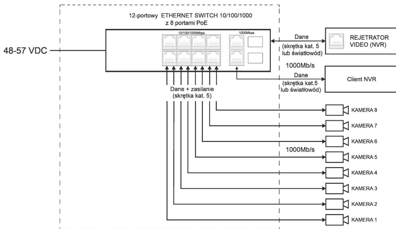
Rys. 1. Schemat blokowy.
