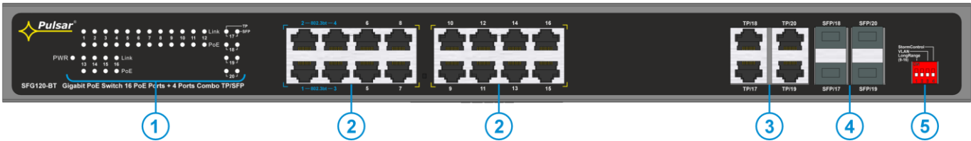
Rys. 2. Panel czołowy switcha.
