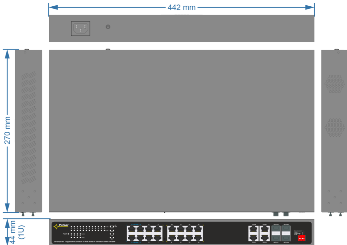
Rys. 4. Widok switch'a.
