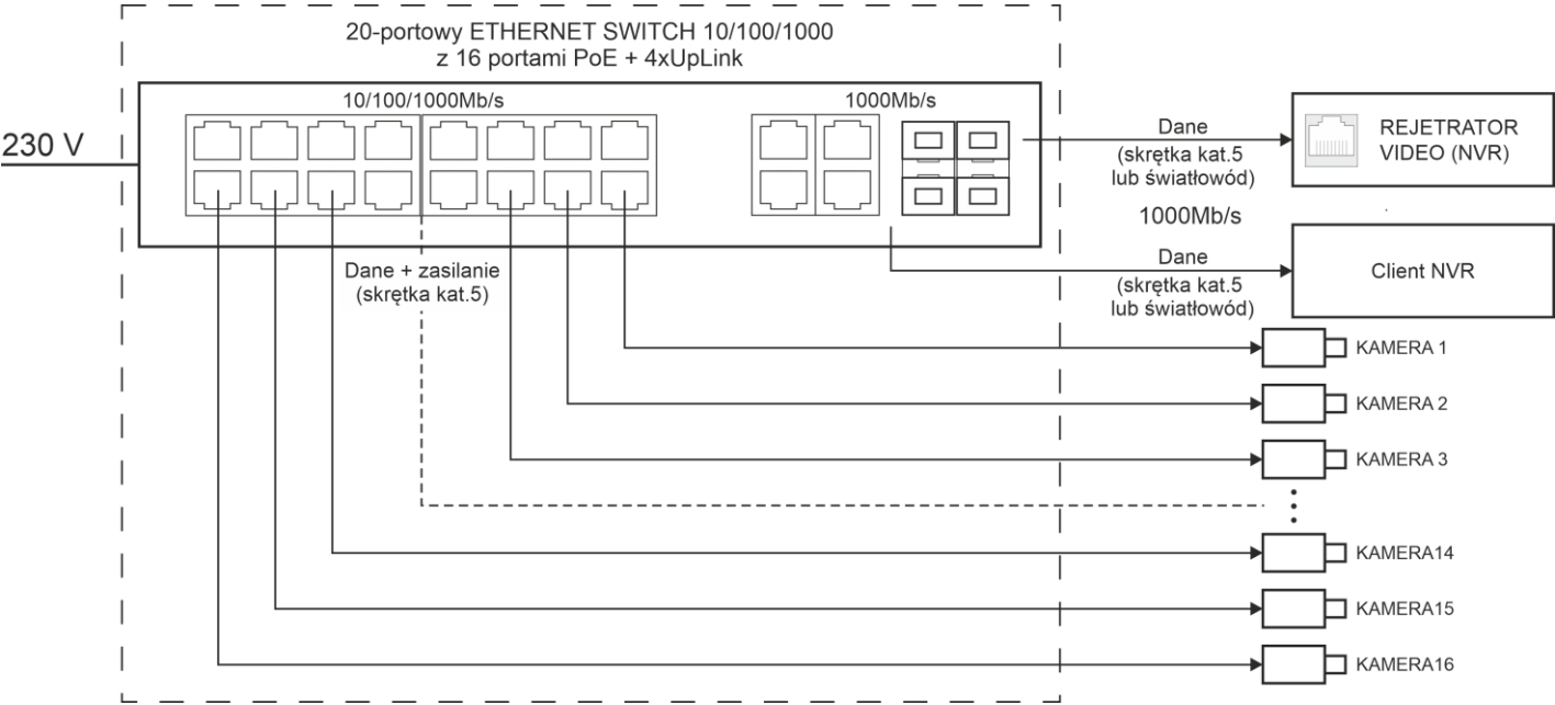
Rys. 1. Schemat blokowy.
