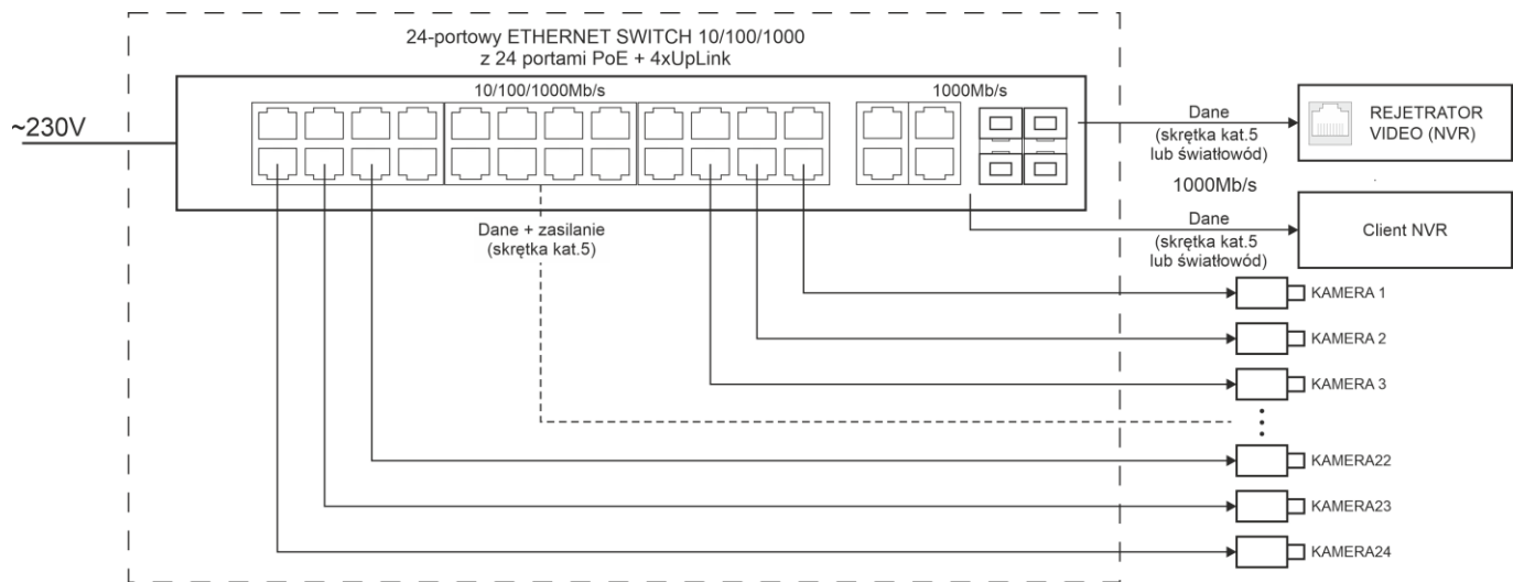
Rys. 1. Schemat blokowy.
