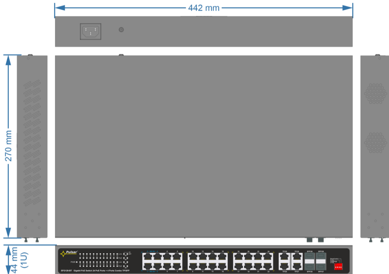
Rys. 4. Widok switch'a.
